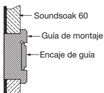
Panel Soundsoak® 60 con guardasillas, guía de montaje y encaje de guía
