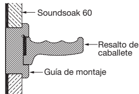
Panel Soundsoak® 60 con guardasillas, guía de montaje con resalto de caballete
