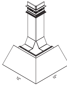
Esquina exterior de plafón a plafón Knife Edge
