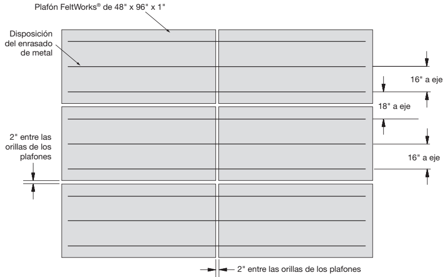
Diseño del enrasado de metal (3 filas por plafón/panel) con una separación recomendada de 2" entre los plafones/paneles para la instalación con tornillo y arandela
