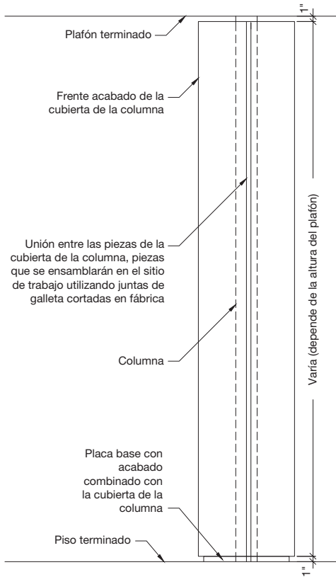
Sección de columna cuadrada
