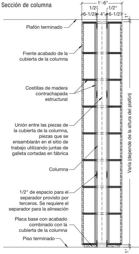
Sección de columna semicircular
