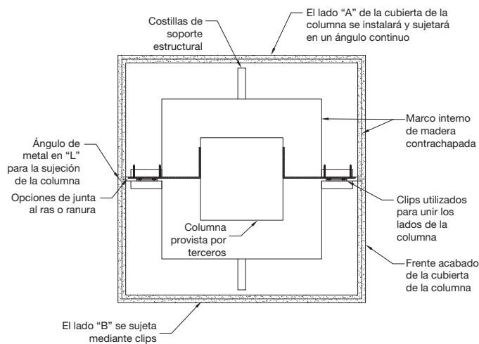
Sección de columna cuadrada
