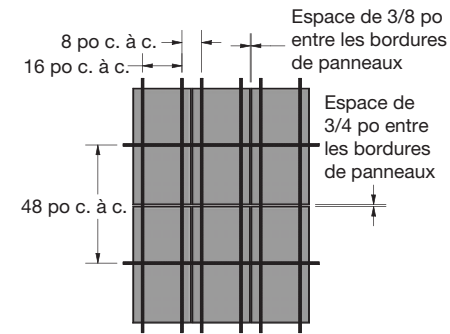
(Fig. 14) Disposition de la suspension de gypse pour panneaux FeltWorks de 24 x 48 po Installation des vis et des rondelles
