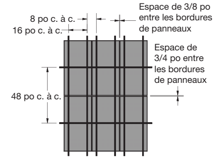
(Fig. 29) Disposition de la suspension de gypse pour panneaux FeltWorks de 24 x 48 po Installation des aimants – non séismique
