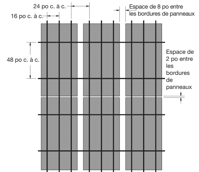
(Fig. 33) Disposition de la suspension de gypse pour panneaux FeltWorks de 48 x 96 po Installation des aimants – sismique
