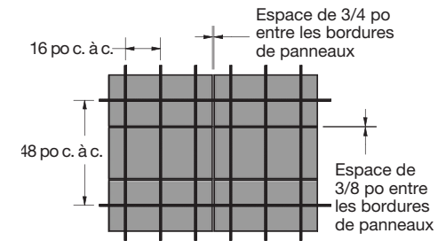
(Fig. 32) Disposition de la suspension de gypse pour panneaux FeltWorks de 24 x 48 po Installation des aimants – sismique
