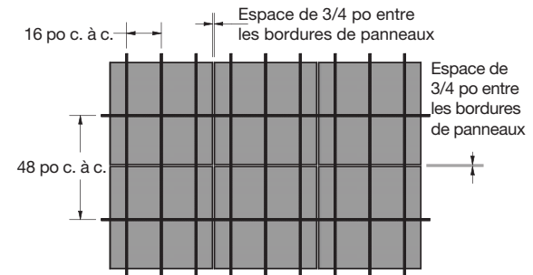
(Fig. 30) Disposition de la suspension de gypse pour panneaux FeltWorks de 48 x 48 po Installation des aimants – non séismique
