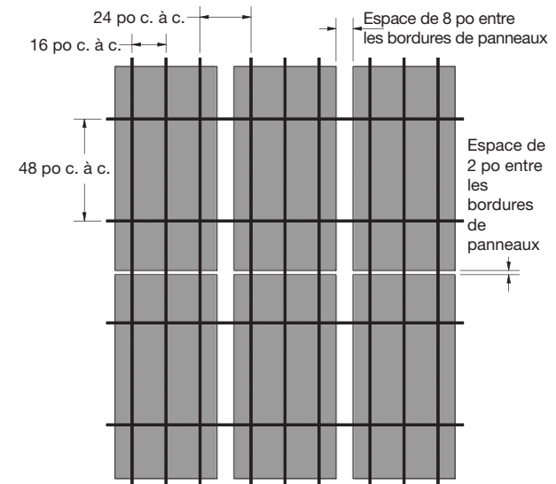
(Fig. 31) Disposition de la suspension de gypse pour panneaux FeltWorks de 48 x 96 po Installation des aimants – non séismique
