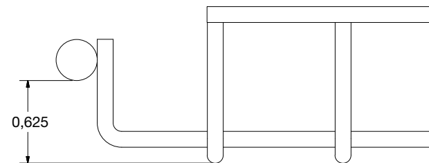
Profil de bordure pour téglulaire soudé
