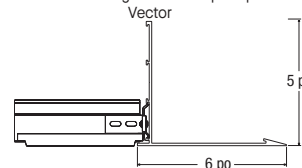
Profil Axiom Knife Edge Tranchant (AXKE5STR)
