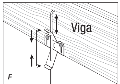
Ganchos para el sistema de suspensión QuickHang
