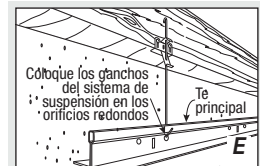
Ganchos para el sistema de suspensión QuickHang
