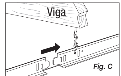
Alambre de colganteo tradicional
