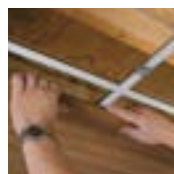
Positionnez les planches; faites glisser et fixez les attaches
